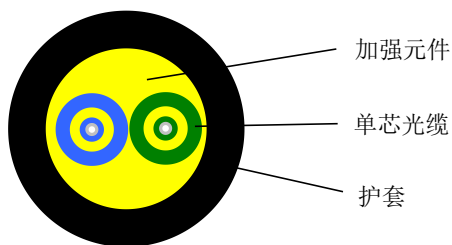
双芯圆形基站光缆 II 型
